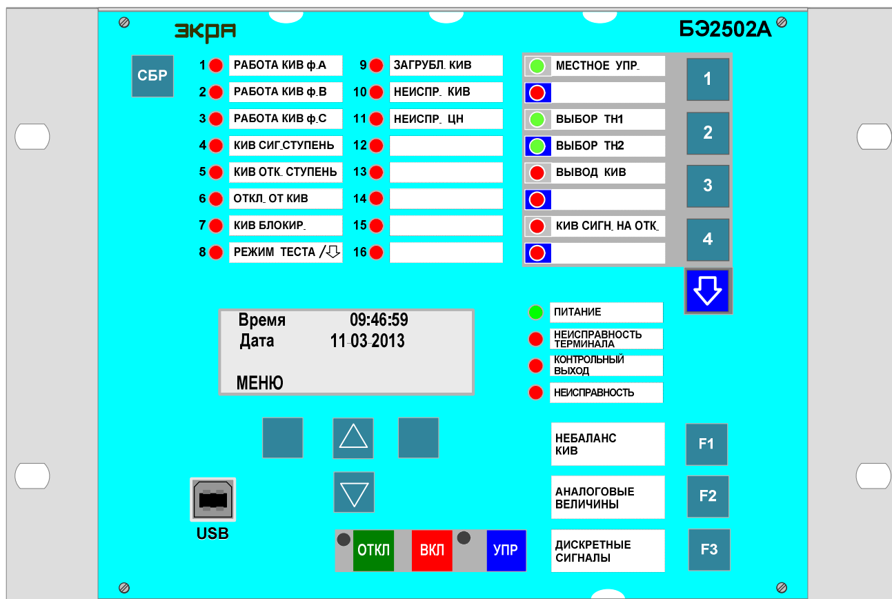
Рисунок 4 – Расположение элементов на лицевой панели терминала БЭ2502А1402
