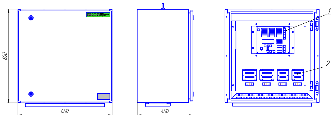
Рисунок 2 – Габаритные, установочные размеры шкафа типа ШНЭ 2114 в кожухе
