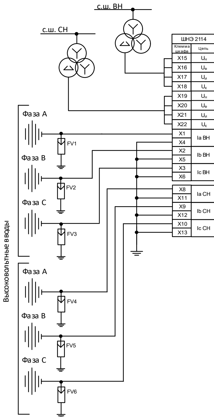
Рисунок 1 – Схема подключения шкафа ШНЭ 2114
