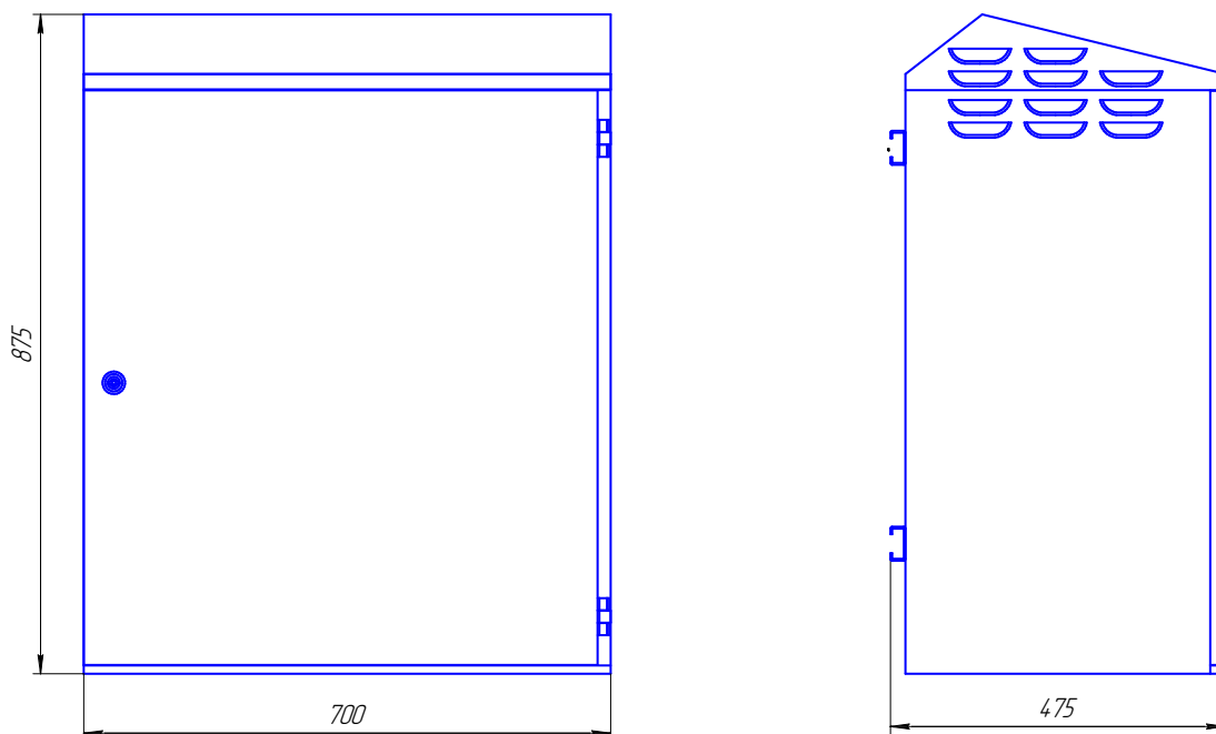
Рисунок 2 – Габаритные, установочные размеры шкафа типа ШНЭ 2114 в кожухе
